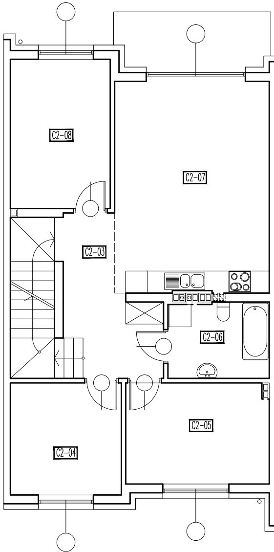
PIĘTRO – budynek C
